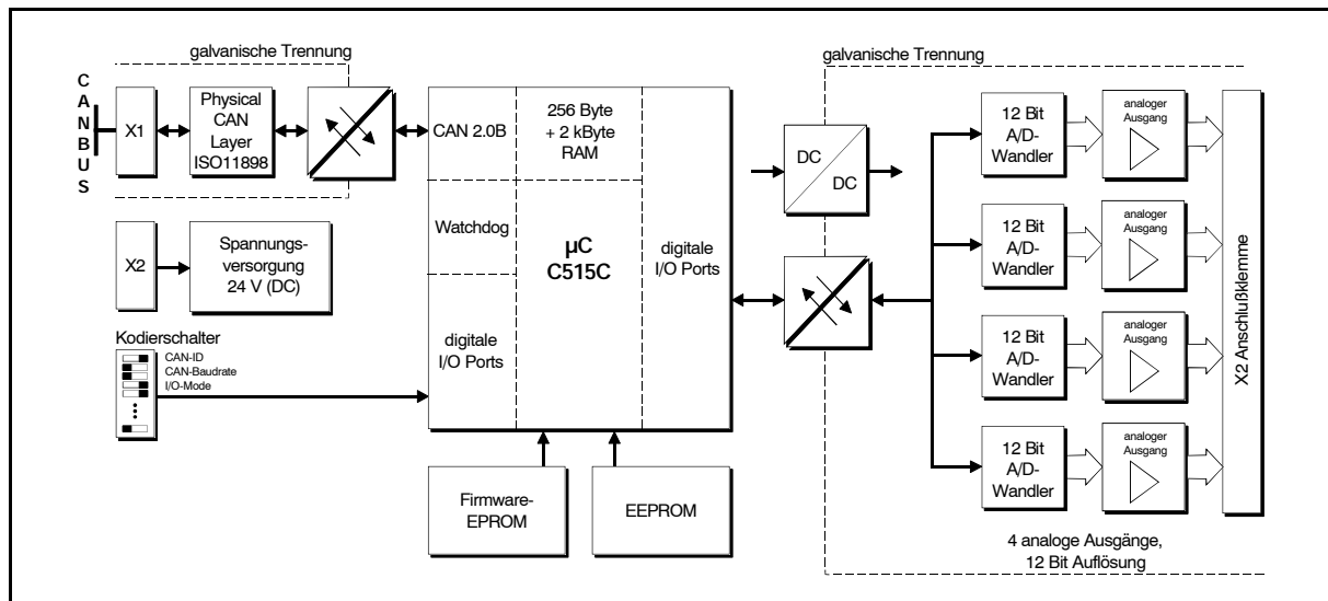
Abb. 1.1.1: Blockschaltbild des CBM-AO4-Moduls
